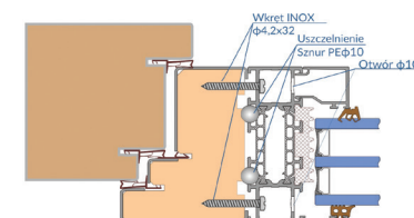
połączenie ościeżnicy z doświetlaniem aluminiowym
